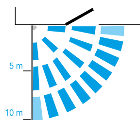
Rivelatore 141-21X - lente volumetrica 90° - portata 10 m
